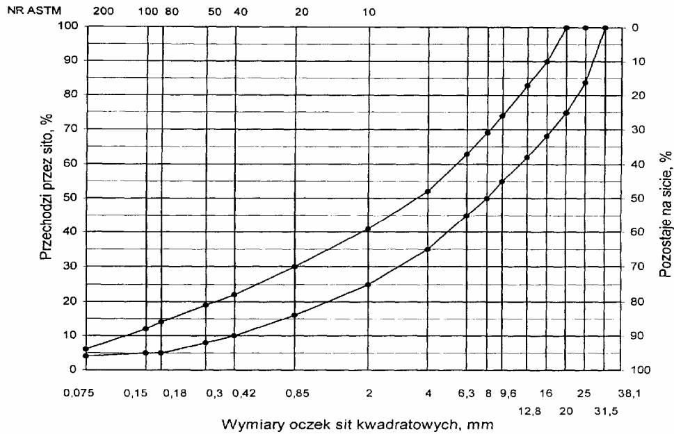
Rys. 11. Krzywe graniczne uziarnienia mieszanki mineralnej BA od 0 do 25 mm do warstwy wiążącej, wyrównawczej
